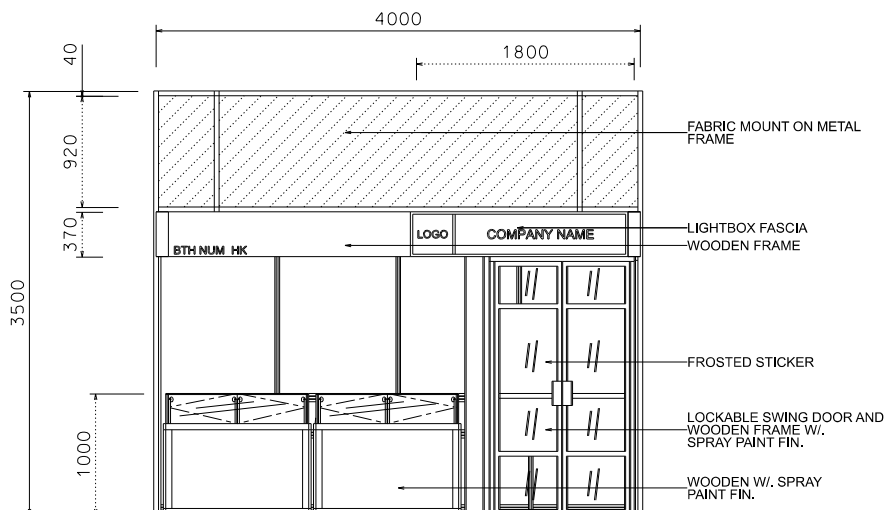
ELEVATION
